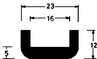
Disegno Scala 1:1
