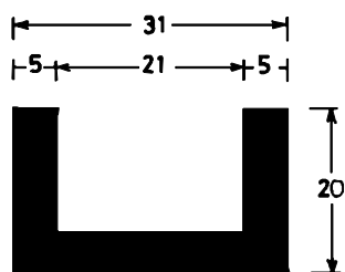
Disegno Scala 1:1
