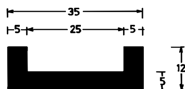
Disegno Scala 1:1
